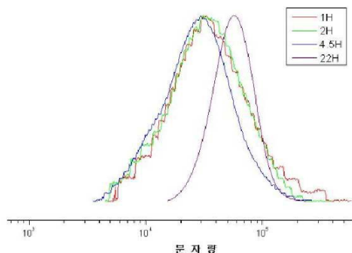
도 1. MDH 입자로부터 그래프팅된 부틸 아크릴레이트의 분자량 분포도. 1시간 후, Mn=26,600; 2시간 후, Mn=24,790; 4시간 후, Mn=21,490; 및 22시간 후 Mn=51,230
