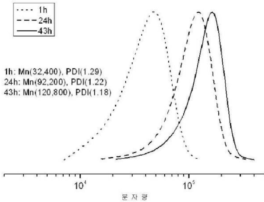
도 6. 개시제가 결합된 MDH로부터 거대 구조의 MMA 중합에 따른 분자량 분포도
